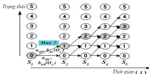
Hình 4: giải thuật Viterbi
