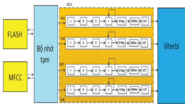
Hình 6: tổng quan các module trong quá trình nhận dạng
