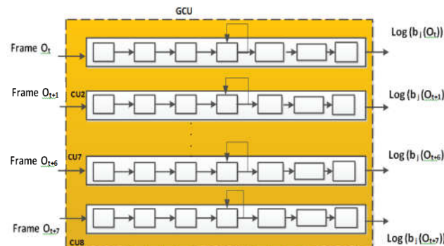
Hình 7: cơ chế tính song song 8 luồng dữ liệu
