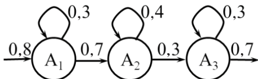
Hình 2: mô hình HMM dạng tiến
