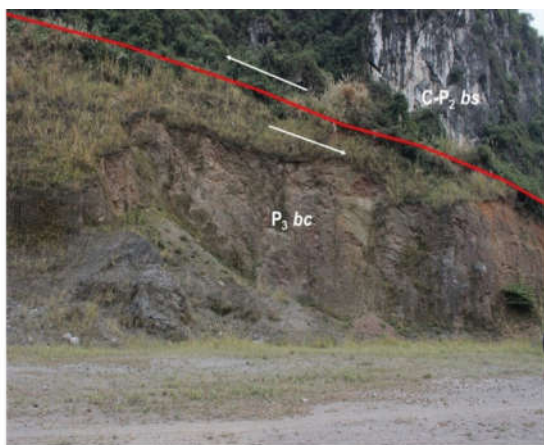
Hình 3: quan hệ chèn lệch giữa đá vôi hệ tầng Bắc Sơn với trầm tích silic hệ tầng Bãi Cháy và hiện tượng uốn nếp đảo đi kèm
