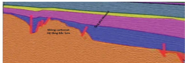
Hình 5: mô hình các bẫy cấu tạo phát triển trên đá móng carbonat tuổi C-P: tầng dưới không có phản xạ địa chấn là tầng móng carbonat, các tầng phản xạ địa chấn được ký hiệu bởi các màu khác nhau bên trên là tầng phủ Đệ Tam, đứt gãy là các đường màu đỏ
