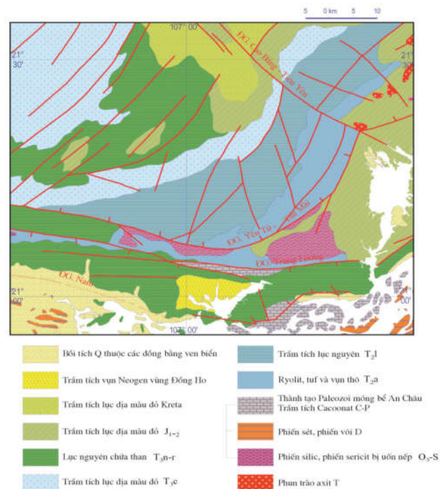
Hình 2: sơ đồ địa chất - kiến tạo giản lược khu vực vùng An Châu theo tài liệu bản đồ địa chất tỷ lệ 1:200.000 từ Lạng Sơn (Hoàng Ngọc Kỳ và nnk, 2000), từ Móng Cái (Nguyễn Công Lượng và nnk, 2000)
