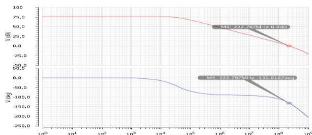
Hình 7: kết quả mô phỏng gain và phase margin của op-amp
