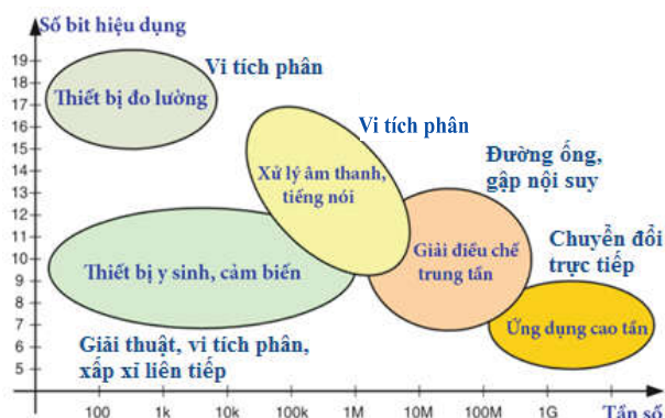
Hình 1: mô hình phân loại kiến trúc ADC theo tần số lấy mẫu và số bit hiệu dụng [2]
