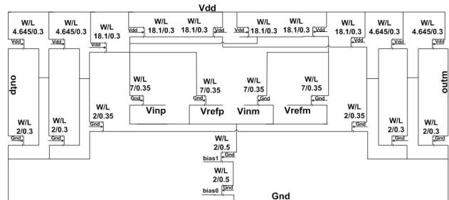
Hình 8: sơ đồ mạch so sánh fully differential two-stage
