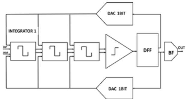
Hình 3: cấu trúc bộ điều biến delta-sigma bậc 3
