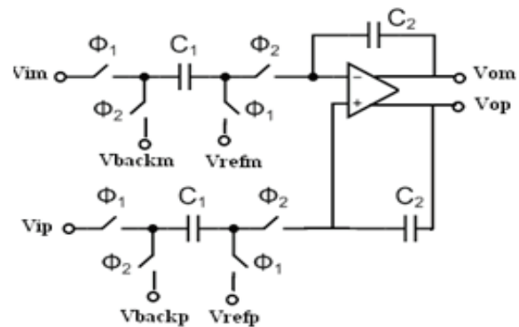
Hình 4: sơ đồ mạch bộ tích phân integrator
