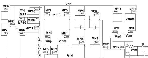
Hình 6: sơ đồ mạch fully differential two-stage op-amp
