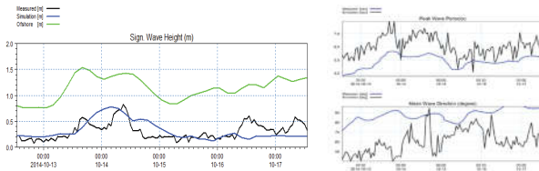
Hình 5: kết quả kiểm định các đặc trưng sóng tính toán với thực đo
