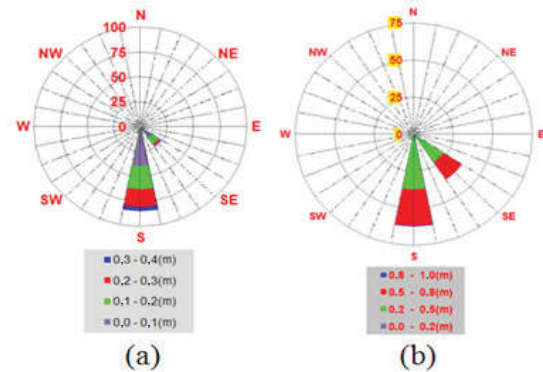
Hình 6: hoa sóng khu vực cửa sông Mã
