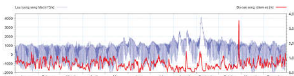
Hình 7: lưu lượng, độ cao sóng tại khu vực cửa sông Mã năm 2012
