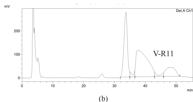
Hình 3: sắc ký đồ HPLC điều chế phân đoạn A4 (a) và C5 (b) Hệ thống HPLC Shizmaszu LC-10AD; cột Discovery HS C18 (250×21,2 mm; 10 μm); phát hiện: UV 190 nm; tốc độ dòng: 15 ml/phút; Pha động: ACN-H 2 O (21:79).
