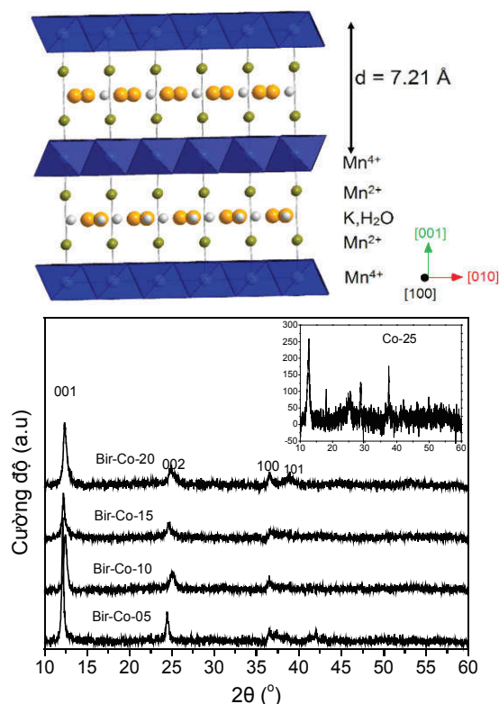
Hình 1: (a) Cấu trúc vật liệu birnessite; (b) Giảm độ nhiễu xạ tia X của các mẫu birnessite pha tạp cobalt
