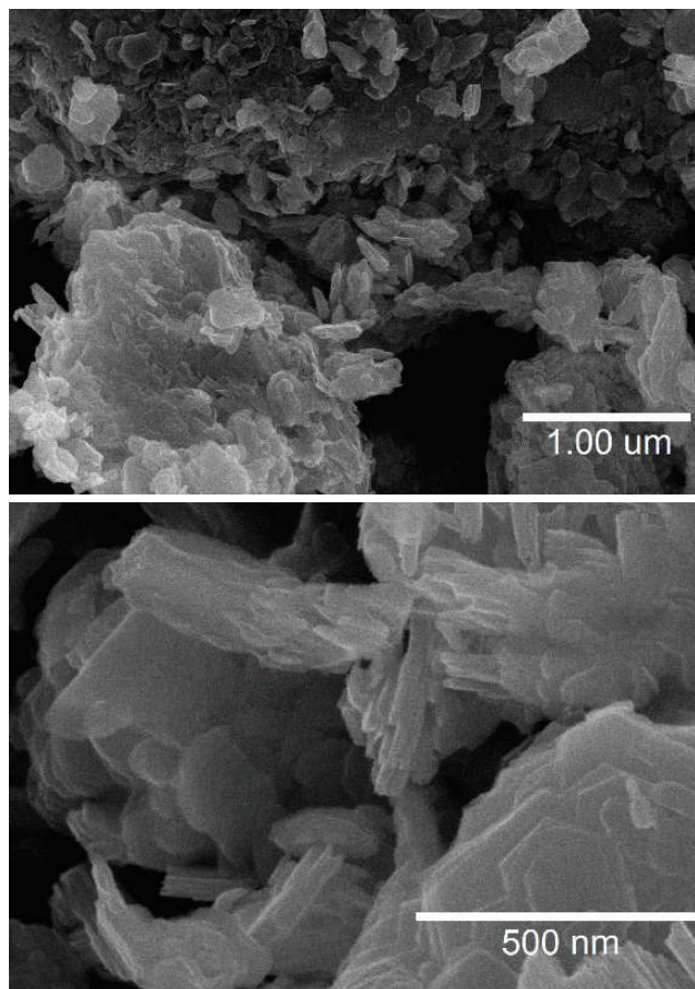
Hình 2: ảnh SEM của mẫu Bir-Co-15
