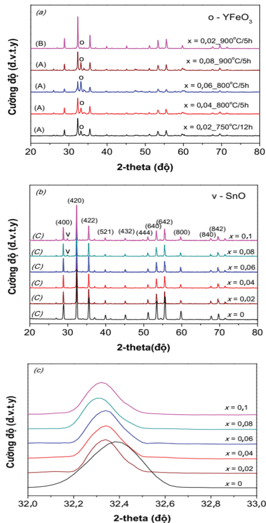
Hình 1. Giản đồ nhiễu xạ tia X của hệ mẫu A và B (a), C (b) và hình phóng đại giản đồ nhiễu xạ tia X tại đỉnh (420) của hệ mẫu C (c).
