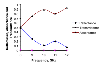
Hình 5: hệ số phản xạ, hấp thụ và truyền qua của sóng điện từ đối với màng sơn PMMA pha trộn 25 wt. % CNTs
