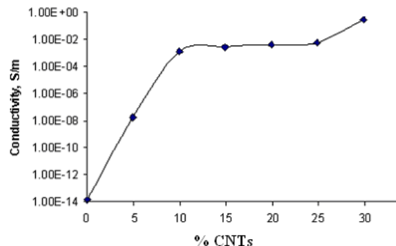
Hình 13: tính dẫn điện của vật liệu composit epoxy/CNTs
