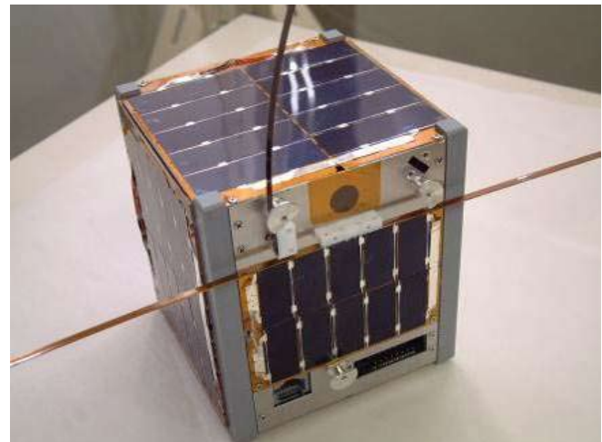
Hình 1: vệ tinh siêu nhỏ XI-IV, phóng năm 2003
