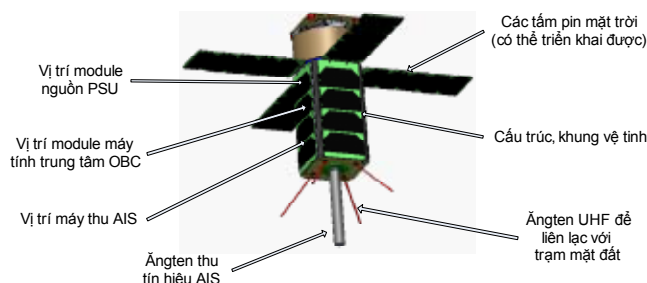
Hình 2: thiết kế của vệ tinh siêu nhỏ 3 kg để theo dõi tàu biển (FSpace) [4]
