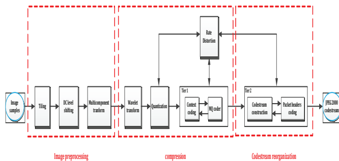
Hình 1: hệ thống nén ảnh JPEG2000
