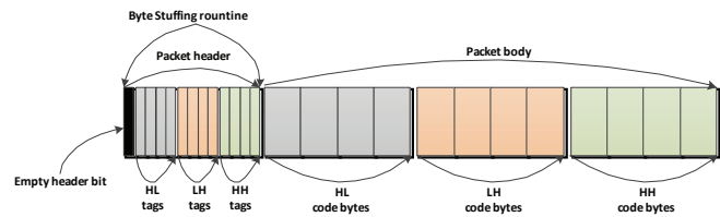
Hình 8: cấu trúc gói [4]
