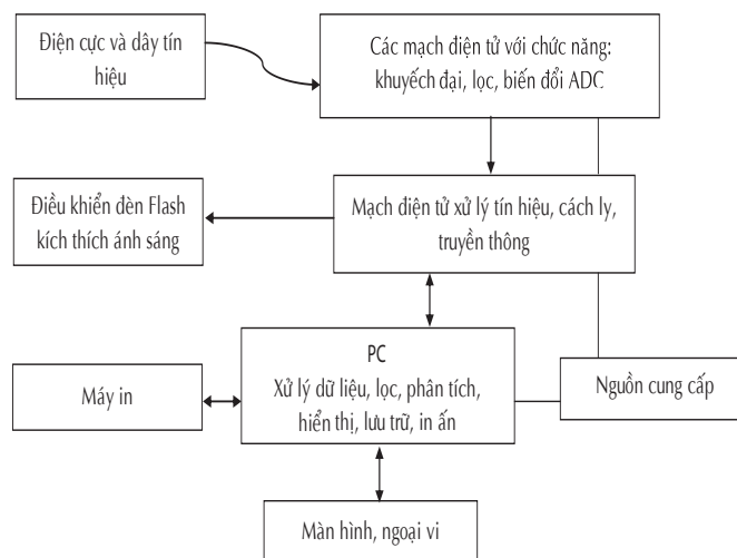
Sơ đồ khối mô tả máy ghi điện não
