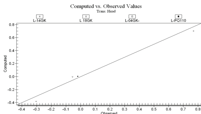
Hình 3: so sánh sai số giữa mực nước quan trắc và tính toán thời điểm tháng 1.2005
