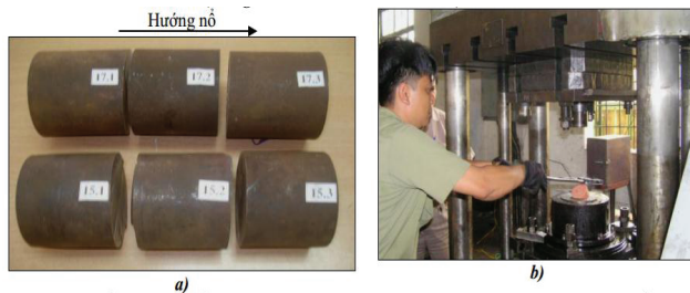
Hình 2: chuẩn bị phôi biến dạng dẻo từ vật liệu bimetal thép C45 và thép WX15 hàn nổ dạng hình trụ (a) và thí nghiệm ép chảy ở trạng thái nóng (b)
