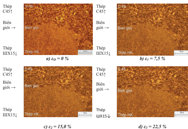
Hình 7: ảnh chụp cấu trúc biên giới 2 lớp mẫu hàn nổ ở chế độ: r = 1,7 ; h = 0,1 ; C = 1,0 : a) chưa qua biến dạng dẻo; b) ép chảy nóng với mức độ biến dạng dẻo lần 1; c) lần 2; d) lần 3
