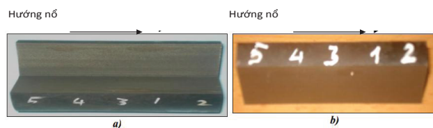
Hình 3: sơ đồ quy ước vị trí cắt lấy mẫu thử phá hủy xác định độ bền bám dính 2 lớp bimetal thép C45 và thép WX15 hàn nổ dạng hình trụ và sau ép chảy nóng
