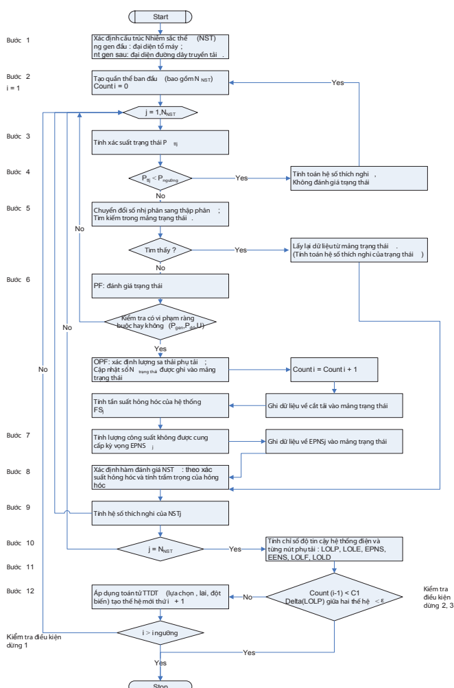
Hình 3: sơ đồ thuật toán đánh giá độ tin cậy hệ thống điện phức tạp bằng phương pháp mô phỏng áp dụng thuật toán di truyền
