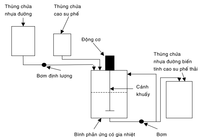
Hình 1: sơ đồ khối quy trình chế tạo nhựa đường biến tính cao su phế thải
