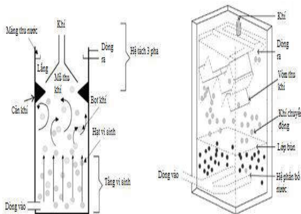
Hình 1: sơ đồ hệ xử lý UASB [15]
