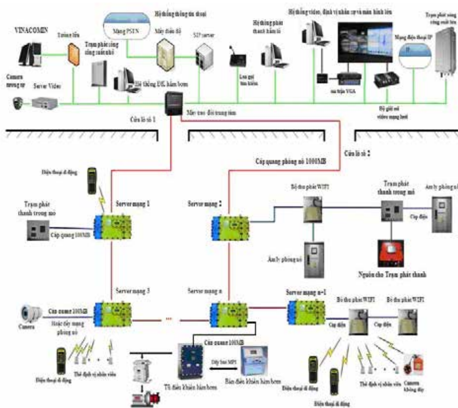
Mô hình tổng thể hệ thống giám sát, điều khiển tập trung hầm lò
